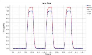
IVT 测试
