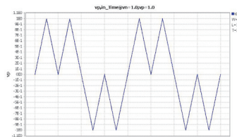
PUND 测试
