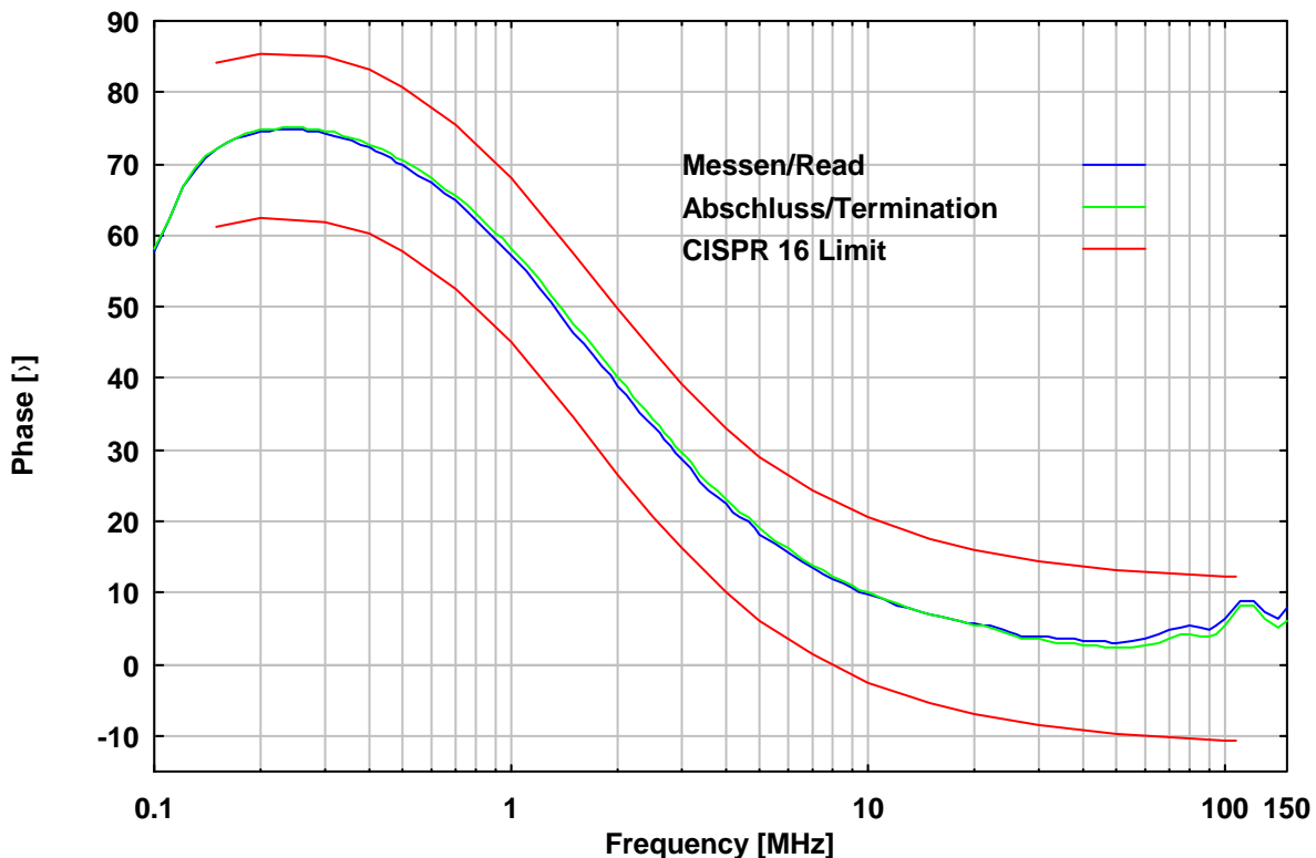
Abb. 6: Phase an den Prüflingsklemmen (Spezialadapter erforderlich), BNC mit 50 \Omega Abschluss, Speiseklemmen offen
