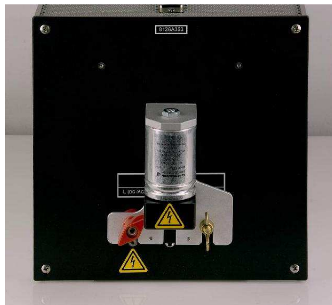
Abb. 3: Befestigung des CAP 10-200 an einer Netznachbildung Fig. 3: CAP 10-200 mounted to a LISN
