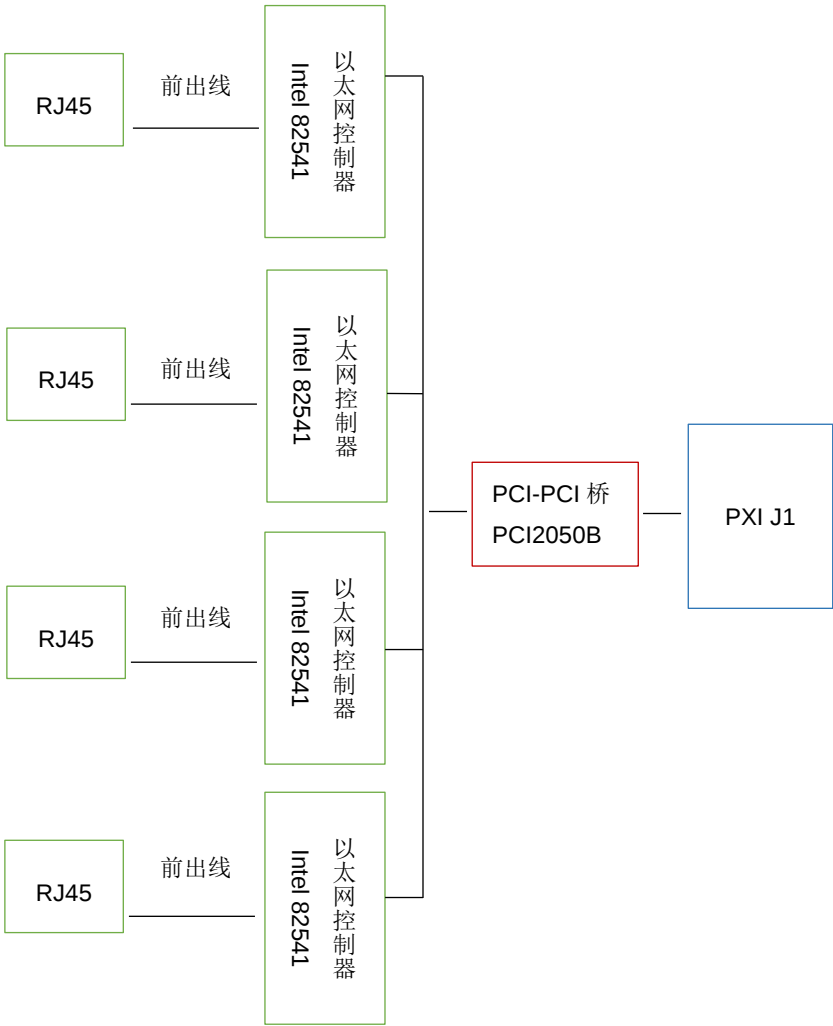
原理框图
