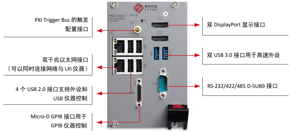
PXle-63977 前面板
