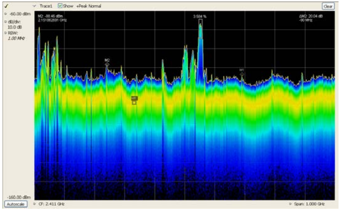
扫频DPX 可以在大于实时带宽的频宽中捕获低概率事件。这里，1 GHz 扫描从未播送信号的天线中扫描 1.9 GHz - 2.9 GHz 的活动。我们看到 1.9 GHz 小区频段中的数字信号，并可以明显看到 2.4 GHz ISM 频段中的重要活动。我们在中心附近的最大信号上同时使用密度测量，显示占用率约为 3.5%。
